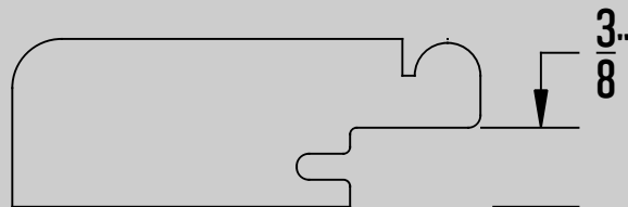
Miter 16 RFG
